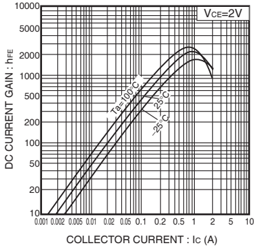
Fig.4 直流電流増幅率-コレクタ電流特性
