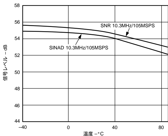
特性13 SINAD / S/N比 対 温度 ( f_{AIN} = 10.3\text{MHz} 、 f_{ENCODE} = 105\text{MSPS} 、 1\text{Vp-p} )
