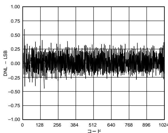
特性18 DNL@80MSPS
