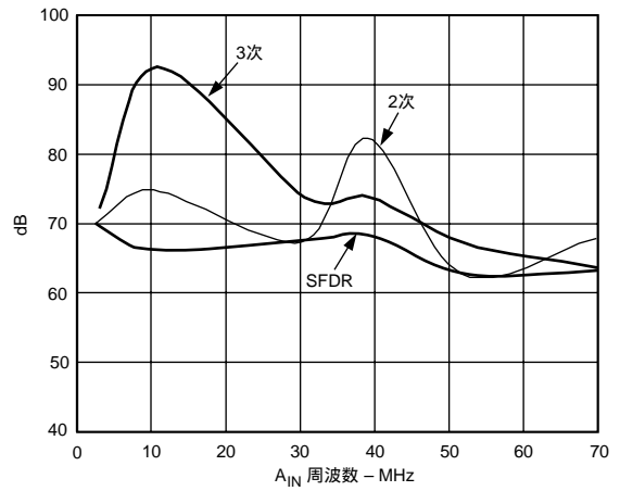
特性5 高調波歪み (2次および3次) およびSFDR 対 A_{IN} 周波数 (1Vp-p, f_s = 105\text{MSPS} )
