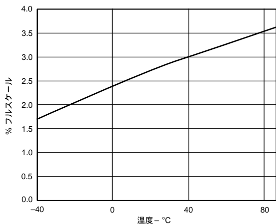
特性14 ADCゲイン 対 温度 (外部1.25Vリファレンス)
