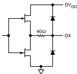
図4 デジタル出力段
