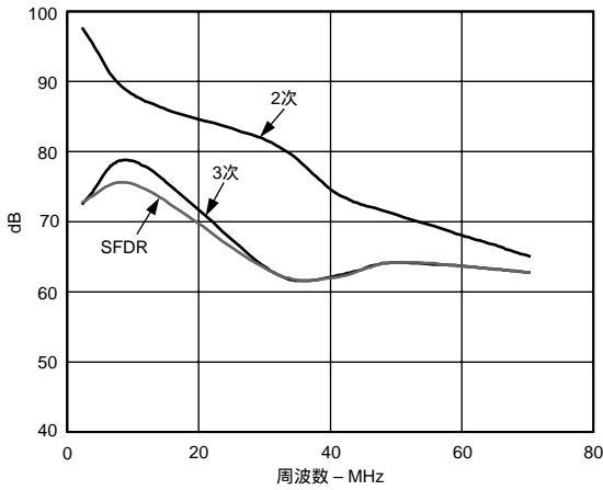
特性7 高調波歪み(2次および3次)およびSFDR 対 A_{IN} 周波数(1Vp-pおよび2Vp-p, f_s = 65\text{MSPS} )
