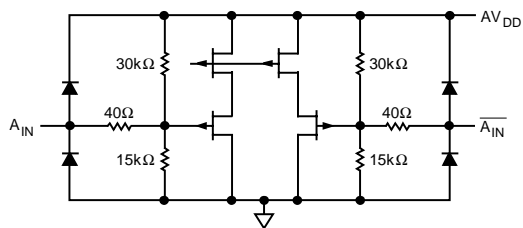
図2 アナログ入力段
