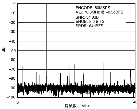
特性2 FFT: f_s = 80\text{MSPS} , f_{IN} = 70\text{MHz} , A_{IN} = -0.5\text{dBFS} , 1Vp-pアナログ入力範囲
