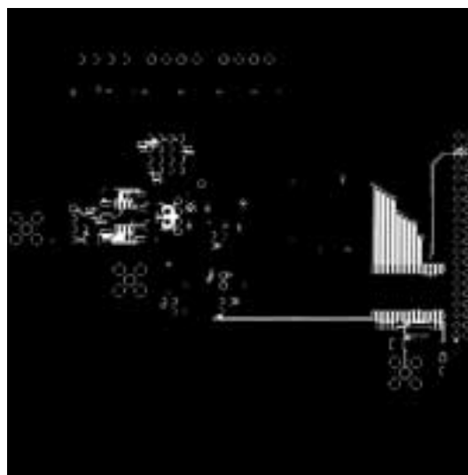
図14 プリント基板底面銅配線面
