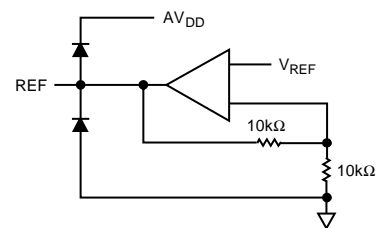
図5 出力に設定されたREF
