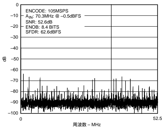
特性3 FFT: f_s = 105\text{MSPS} , f_{IN} = 70\text{MHz} (1Vp-p)
