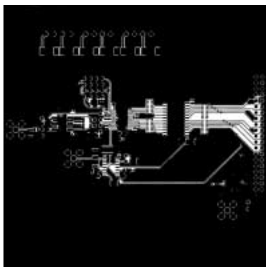
図12 プリント基板上面銅配線面
