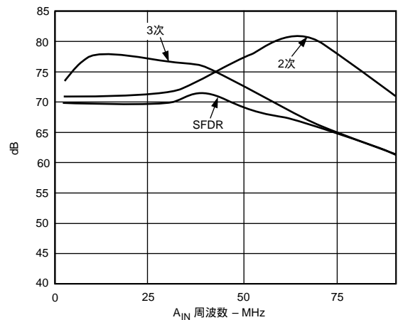
特性6 高調波歪み (2次および3次) およびSFDR 対 A_{IN} 周波数 (2Vp-p, f_s = 80\text{MSPS} )
