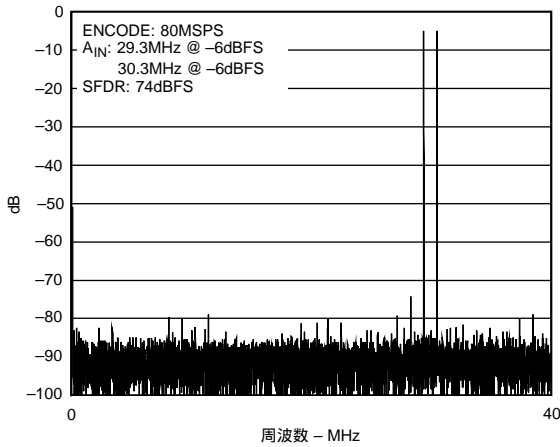
特性8 2トーン相互変調歪み(29.3MHz、30.3MHz、1Vp-p、 f_s = 80\text{MSPS} )
