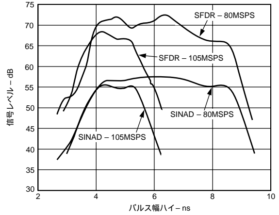
特性11 SINADおよびSFDR 対 エンコード・パルス幅ハイ(1Vp-p)
