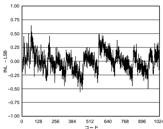
特性17 INL@80MSPS
