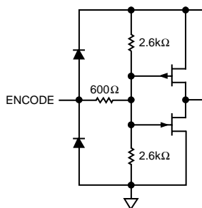
図3 エンコード入力
