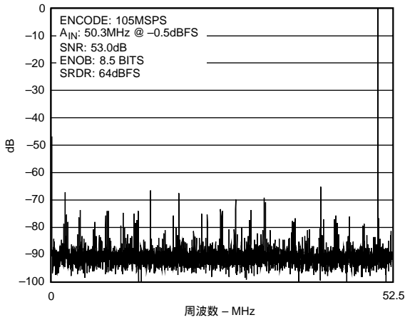
特性1 FFT: f_s = 105\text{MSPS} , f_{IN} = \sim 50.3\text{MHz} , A_{IN} = -0.5\text{dBFS} , 差動、1Vp-pアナログ入力範囲
