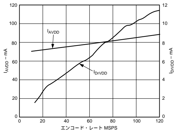
特性12 I_{AVDD} および I_{DrVDD} 対 エンコード・レート ( f_{AIN} = 10.3\text{MHz} , -0.5 dBFS、および -3dBFS) デジタル出力における C_{LOAD} \sim 7\text{pF}
