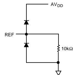
図6 入力に設定されたREF
