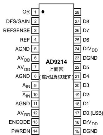
AD9214 ピン配置
