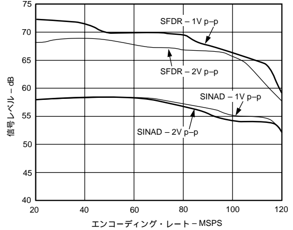
特性10 SINADおよびSFDR 対 エンコード・レート ( f_{IN} = 10.3\text{MHz} , 1Vp-pおよび2Vp-p)
