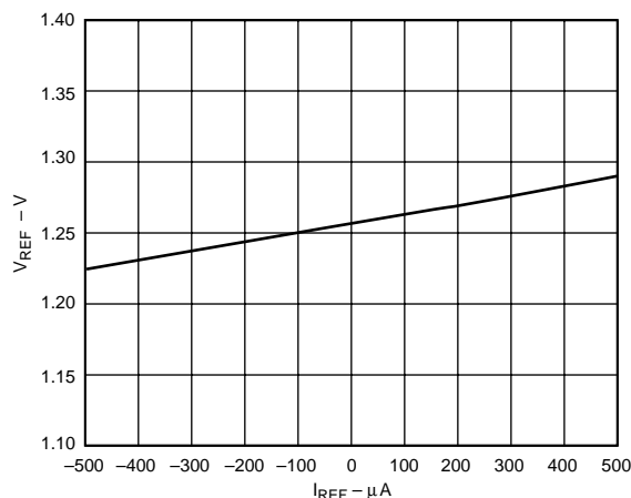
特性16 ADCリファレンス 対 電流負荷
