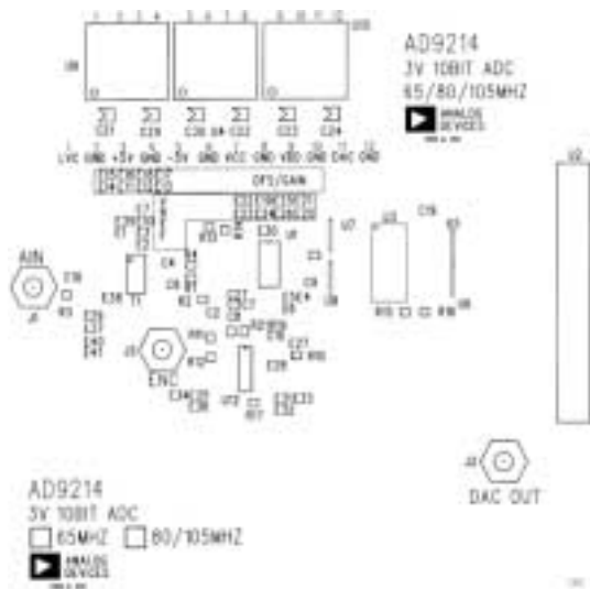
図11 プリント基板上面シルク・スクリーン
