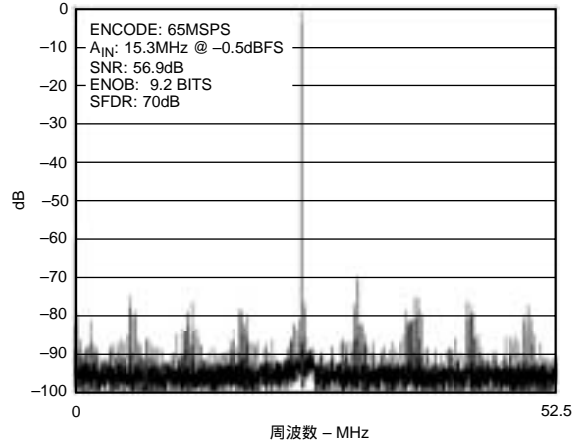
特性4 FFT: f_s = 65\text{MSPS} , f_{IN} = 15.3\text{MHz} (2Vp-p), AD8138で A_{IN} をドライブ
