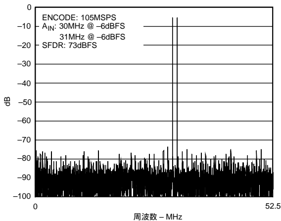
特性9 2トーン相互変調歪み(30MHzおよび31MHz、1Vp-p、 f_s = 105\text{MSPS} )
