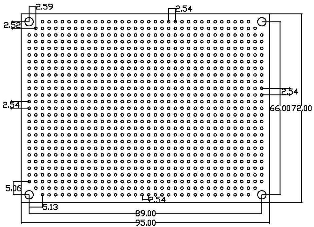
치수도 2
