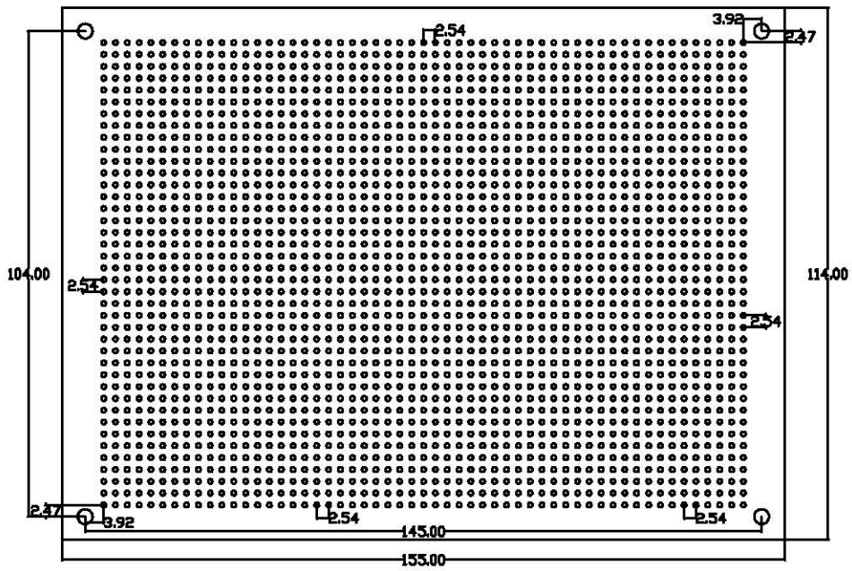
치수도 2
