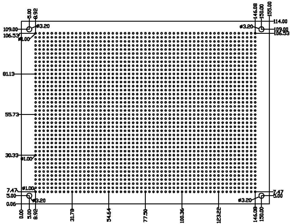
치수도 1
