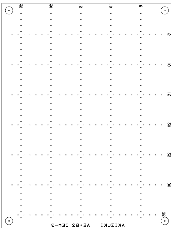
AE-B2_CEM-3 (H21.09.07) 部品面シルク (半田面視)
