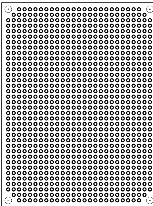
AE-B2_TH (H21.09.07) 部品面パターン (半田面視)
