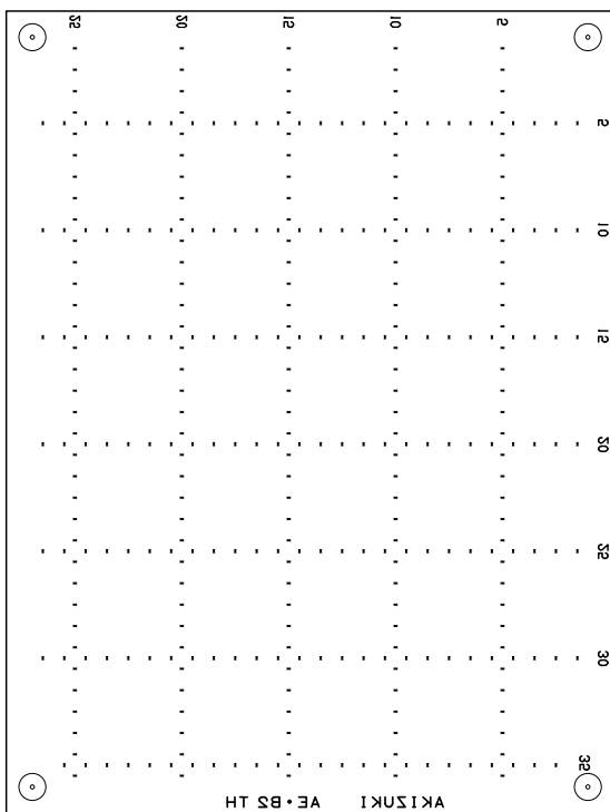
AE-B2_TH (H21.09.07) 部品面シルク (半田面視)
