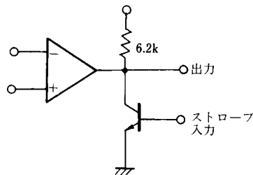
出力ストロープ回路
