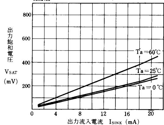
出力流入電流対出力飽和電圧特性例 ( V^+ = 5\text{ V} ) NJM2403
