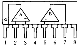
NJM2903L/2403L
