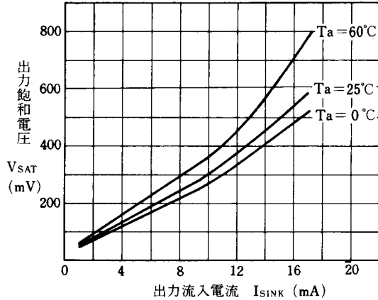
出力流入電流対出力飽和電圧特性例 ( V^+ = 5\text{ V} ) NJM2903
