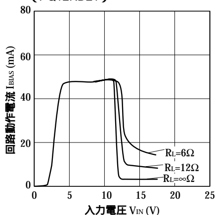
図 19 回路動作電流 - 入力電圧特性 (PQ12RD21)
