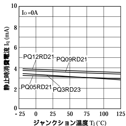
図 21 静止時消費電流 - ジャンクション温度特性
