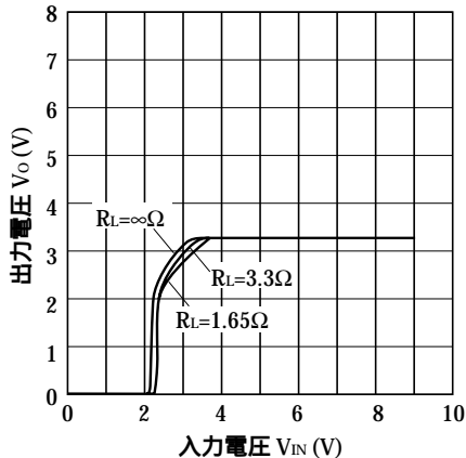
図 12 出力電圧 - 入力電圧特性 (PQ3RD23)
