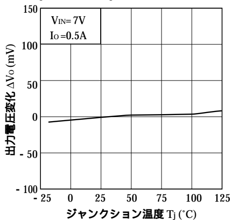
図9 出力電圧変化 - ジャンクション温度特性 (PQ05RD21)
