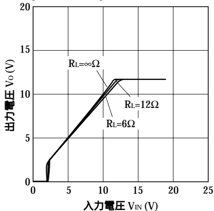
図 15 出力電圧 - 入力電圧特性 (PQ12RD21)
