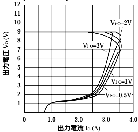
図6 過電流保護特性 (代表値) (PQ09RD21)
