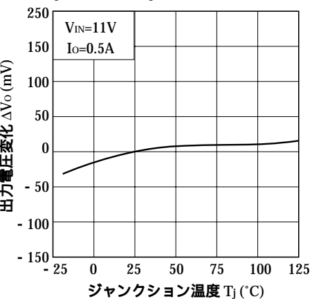
図10 出力電圧変化 - ジャンクション温度特性 (PQ09RD21)
