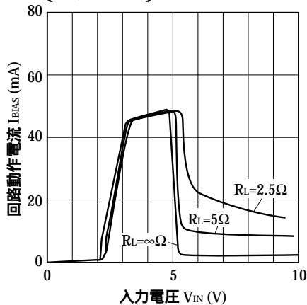
図 17 回路動作電流 - 入力電圧特性 (PQ05RD21)
