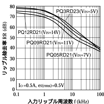
図 22 リプル除去率 - 入力リップル周波数特性
