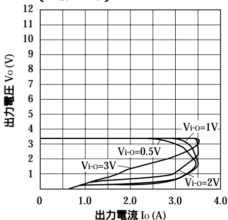
図4 過電流保護特性 (代表値) (PQ3RD23)
