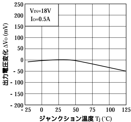
図 11 出力電圧変化 - ジャンクション温度特性 (PQ12RD21)
