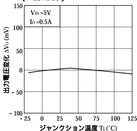
図8 出力電圧変化 - ジャンクション温度特性 (PQ3RD23)
