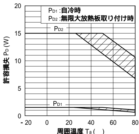
図3 許容損失低減曲線
