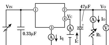
図1 レギュレータ標準測定回路
