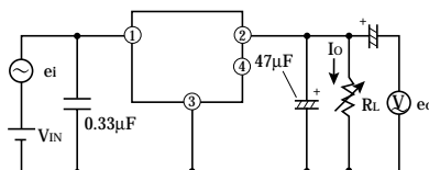
図2 リップル除去率測定回路
