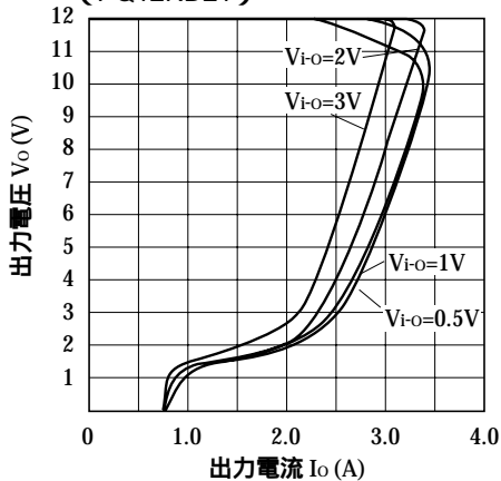
図7 過電流保護特性 (代表値) (PQ12RD21)
