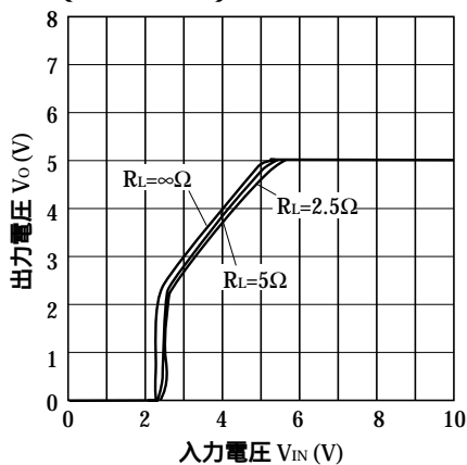
図 13 出力電圧 - 入力電圧特性 (PQ05RD21)
