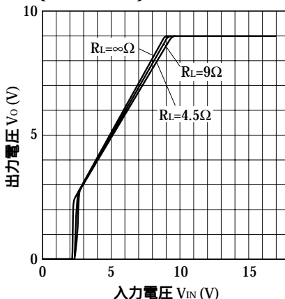
図 14 出力電圧 - 入力電圧特性 (PQ09RD21)
