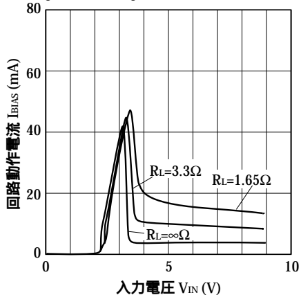
図 16 回路動作電流 - 入力電圧特性 (PQ3RD23)
