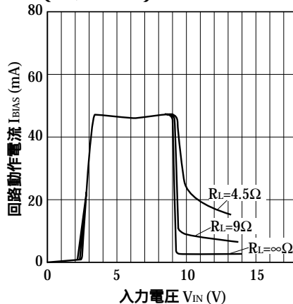
図 18 回路動作電流 - 入力電圧特性 (PQ09RD21)
