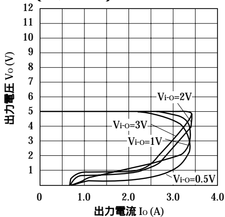
図5 過電流保護特性 (代表値) (PQ05RD21)
