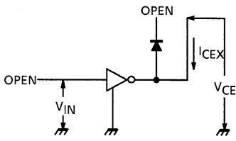
1. I_{CEX}
